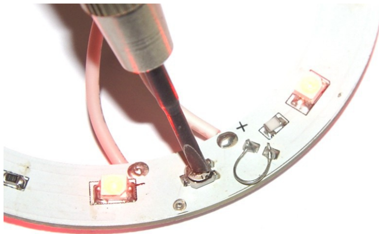
"Abschalten" LEDs Unterseite, "Turn off" bottom LEDs
