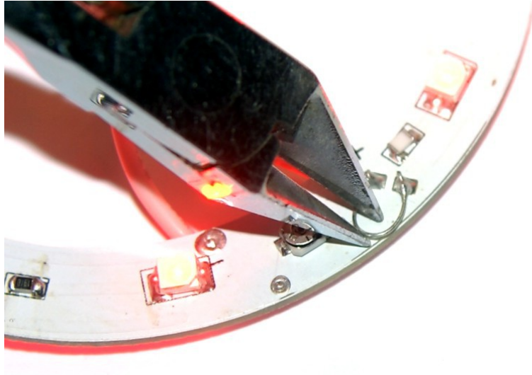
"Abschalten" LEDs Unterseite, "Turn off" bottom LEDs
